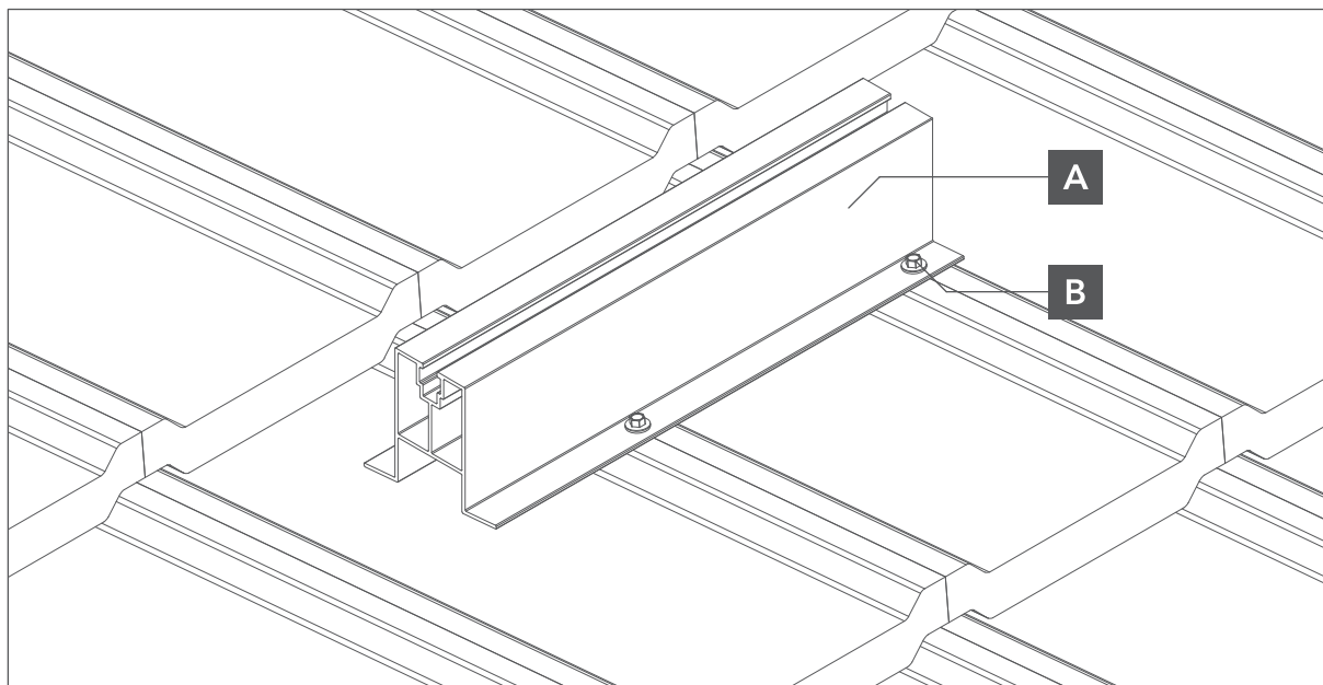
Rys. 4. Mocowanie mostków trapezowych
