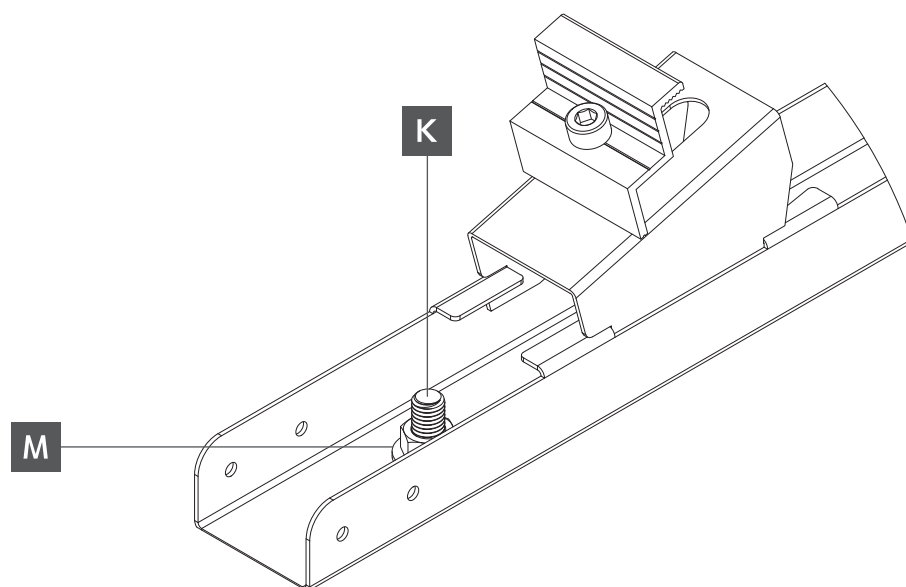
SZCZEGÓŁ A
